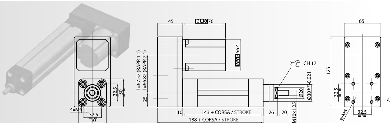
MOTORE / MOTOR STEPPER
