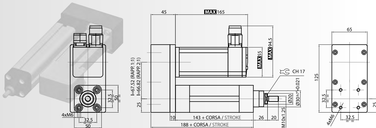
MOTORE / MOTOR BRUSHLESS
